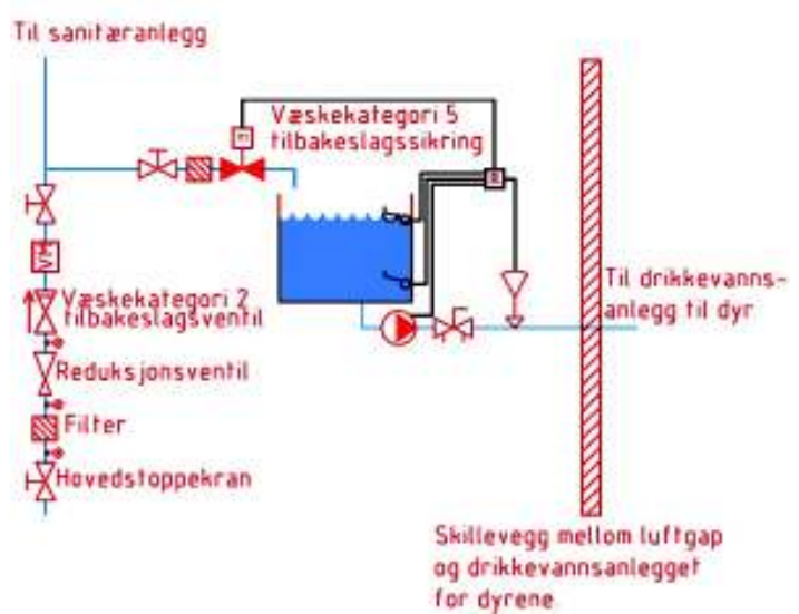
Prinsippskisse for drikkevannsanlegg til dyr
