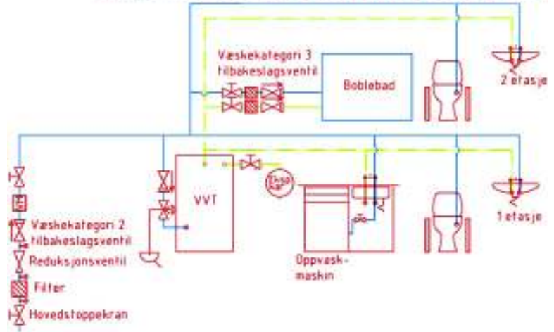
Prinsippskisse for boblebad med påfylling under vannspeil
