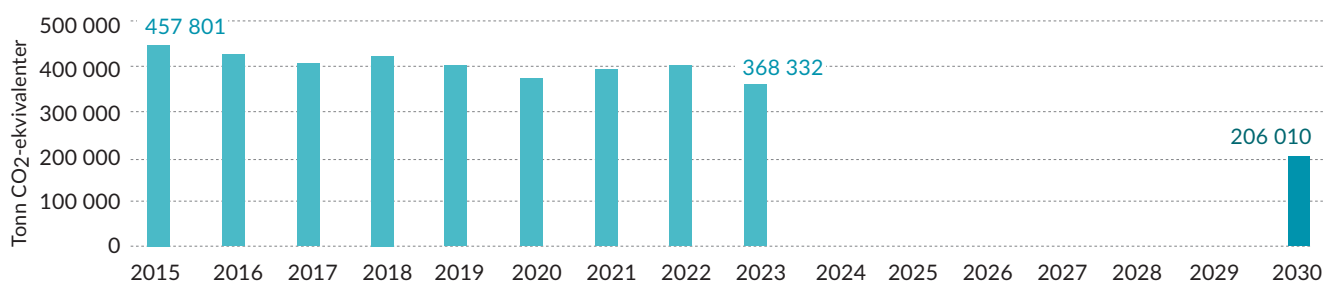
Figur 4: Direkte klimagassutslipp i Kristiansand og mål om 55 prosent reduksjon i 2030
