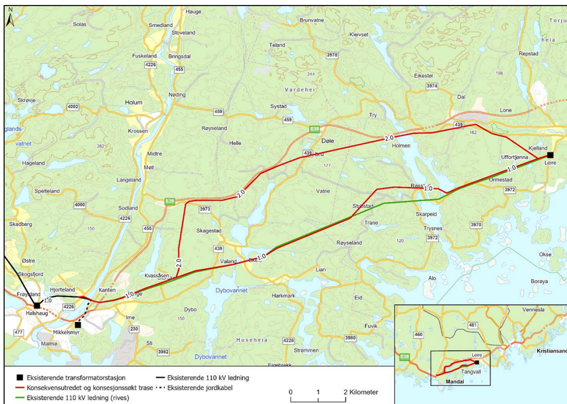
Figur 1 Oversiktskart over omsøkte traseer vist med rød strek. Grønn strek er dagens ledningstrase.
