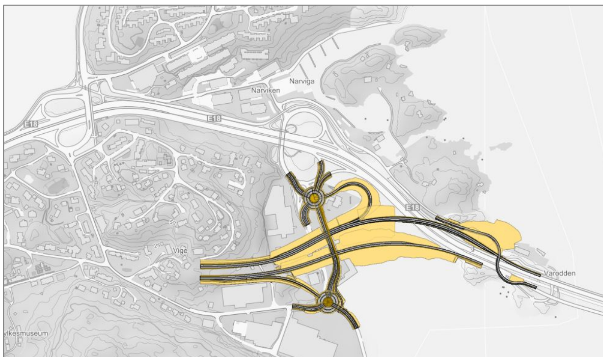
Figur 4-3: Kryssalternativ VS2 i Vige. Krysskonseptet går ut på at ny Ytre ringvei gafler av fra eksisterende E18 og går inn i tunnel sør for E18 etter å ha krysset over Vigebukta på fylling.
