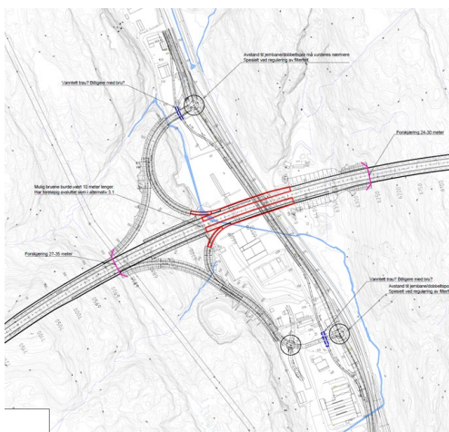
Figur 3-3: Oversikt over kryssløsningene i Dalane som var gjenstand for vurdering og valg.
