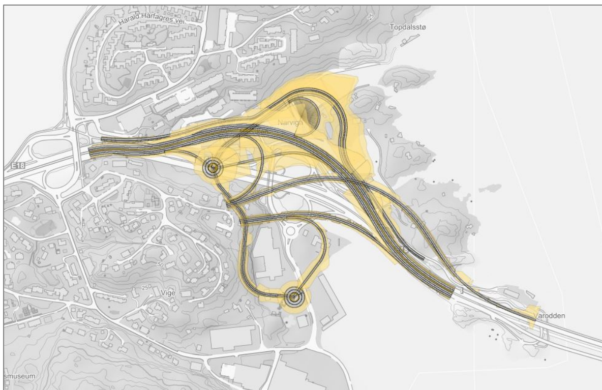
Figur 4-2: Kryssalternativ VS1 i Vigje. Krysskonseptet går ut på at ny Ytre ringvei gafler av fra eksisterende E18 og går inn i tunnel i sonen like sør for E18. Løsningen innebærer utfylling i Narvika og betydelig omlegging av dagens E18 og sykkelspressvei.
