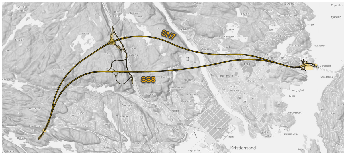
Figur 5-1: Oversiktsfigur tunnelalternativ SN7 (kryss i dagen i Dalane) og SS8 (kryss i berg i Dalane).
