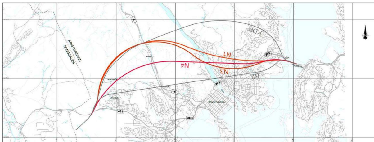
Figur 1-7: Figuren viser et utvalg av mulige veilinjer som ble identifisert i verdiøkingsprosessen.
