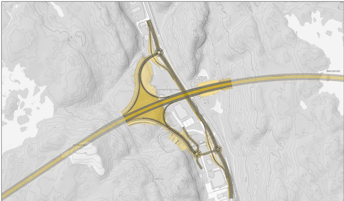
Figur 5-2: Kryssløsning DN, nord i Dalane. Det meste av skissert kryss ligger i dagsone, men tre av fire fartsendingsfelt strekker seg inn i tunnel. Krysset betinger etablering av motorvei på bro over rv. 9, Sørlandsbanen og deler av kollektivterminal. På rv. 9 etableres to nye rundkjøringer med armer til ringveien. Mellom rundkjøringene må rv. 9 oppgraderes til 4-felt. Kryssløsningen er å betrakte som en videreutvikling av anbefalt kryssløsning i KDP.
