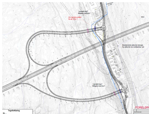
Figur 3-3: Oversikt over kryssløsningene i Dalane som var gjenstand for vurdering og valg.
