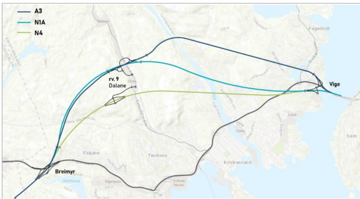
Figur 1-8: Kost/nytte-vurderinger av veilinjene vist i figur 1-7 resulterte i veilinjene illustrert i denne figuren.
