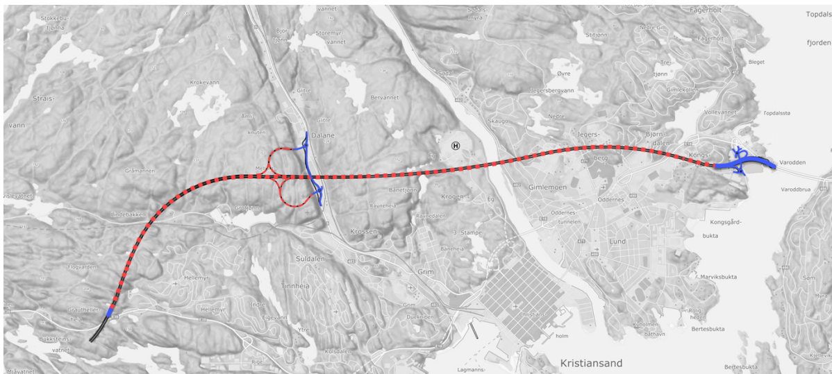
Kartskisse for alternativ SS8. Basert på vurderingene har Nye Veier valgt å fremme dette alternativet for videre detaljering og regulering. Blå heltrukken linje viser veitrasé i dagen, mens stiplet rød linje illustrerer tunnel.
