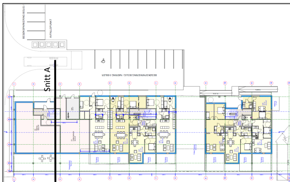
Plantegning som viser snitt gjennom ny bebyggelse.
