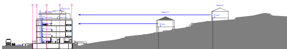
Snitt A-A viser høydeforhold mellom ny bebyggelse og eiendommer i Bliksheia 13 og 15.
