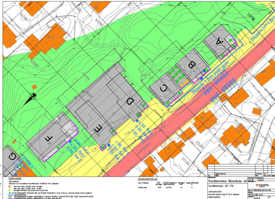
Utsnitt fra støysonekart for Vardåsveien som viser foreslåtte støyruserende tiltak.
